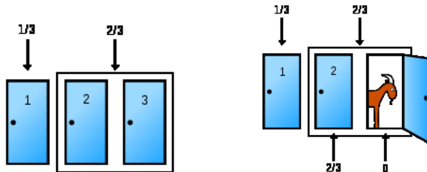
Slika 2. Raspodjela vjerojatnosti za osvajanje auta (uz pretpostavku da je natjecatelj prvotno izabrao vrata 1, a voditelj kviza otvorio vrata 3).
